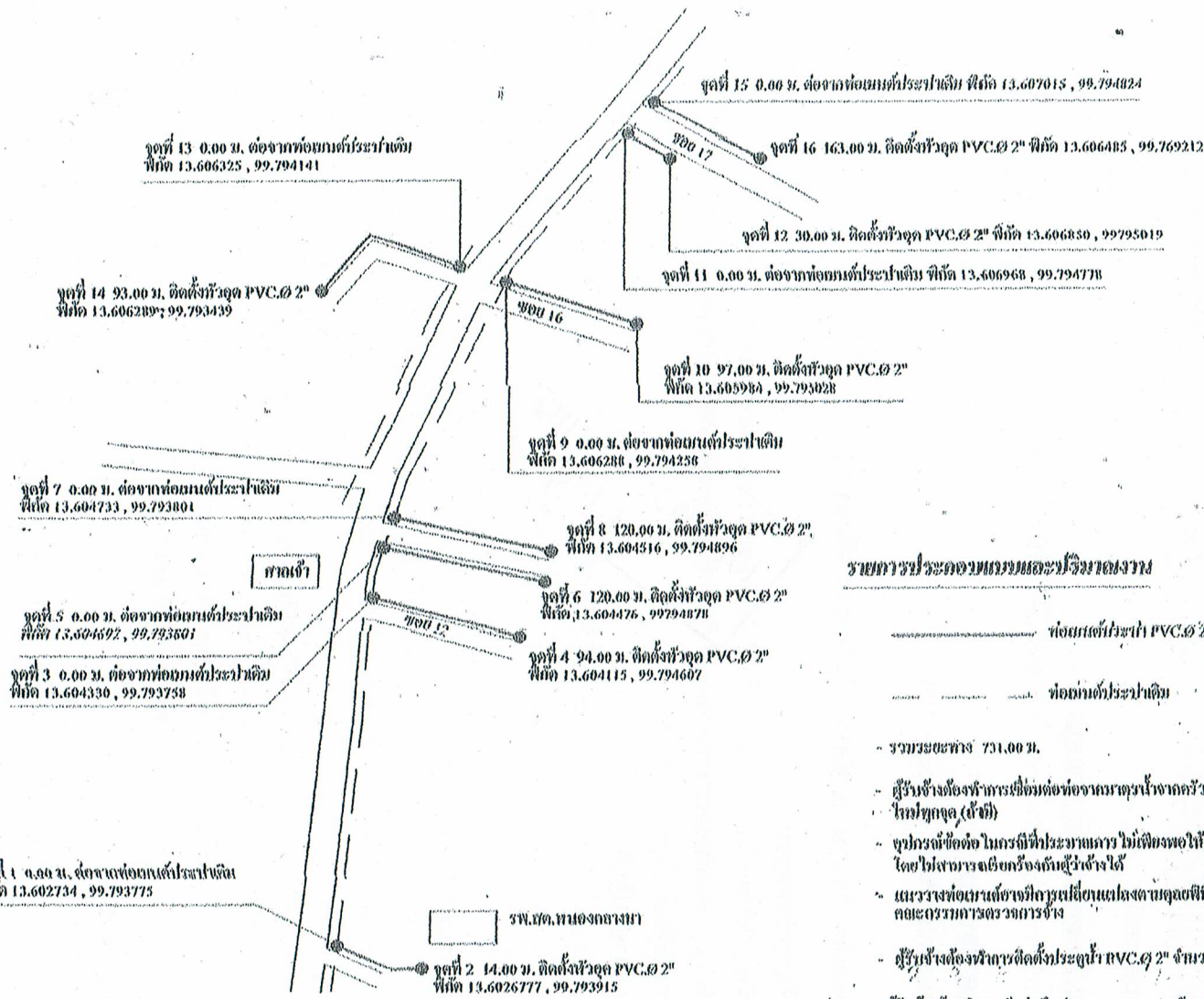
รูปแนวขยายท่อเมนที่ส่งน้ำประปาหมู่ที่ 3 ตำบลหนองกลางนา
